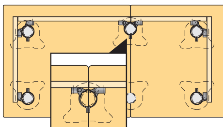
Zwei Tischplatten "auf Stoß" montiert Two table tops mounted side by side Deux plateaux de table montés "en bout" Due piani congiunti Dos mesas montadas "juntas" Dwie płyty stołowe montowane "na styk" Dois tampos de mesa montados "com junta" Två bordsplattor monterade kant i kant To bordplader monteret ved siden af hinanden "Kenarları bitişik" monte edilmiş iki masa tablası Δύο πλάκες επιφανείας τραπεζιού συναρμολογημένες "μέσω ώθησης" Dvě desky stolu montované "na sraz" Két asztallapot egymáshoz illesztve szerelve Две деки стола монтированы "встык"
