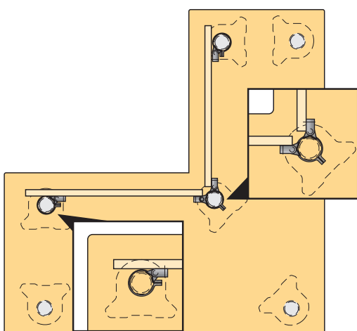
Tisch mit zwei Blenden Table with two modesty panels Table avec deux voiles de fond Piano con due paragambe Mesa con dos paneles Stół z 2 blendami Mesa com dois painéis Bord med två sargar Bord med to kanter İki kordonlu masa Τραπέζι με δύο πλαίσια στήριξης stůl se dvěma clonami asztal két borítással стол с двумя панелями
