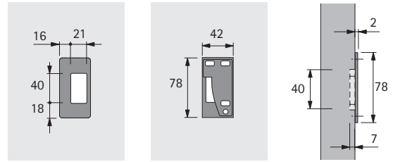
Schließblech Strike plate
