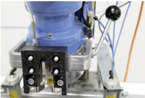
Abb. 26: Einpressmatrize
