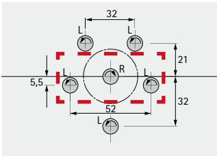
Abb. 28: Bohrbild
