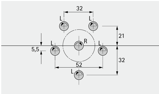
Abb. 17: Bohrbild
