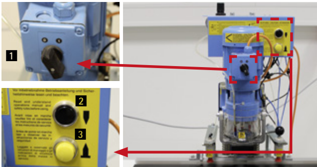
Abb. 5: Bedienelemente am Bohr- und Einpressautomaten
