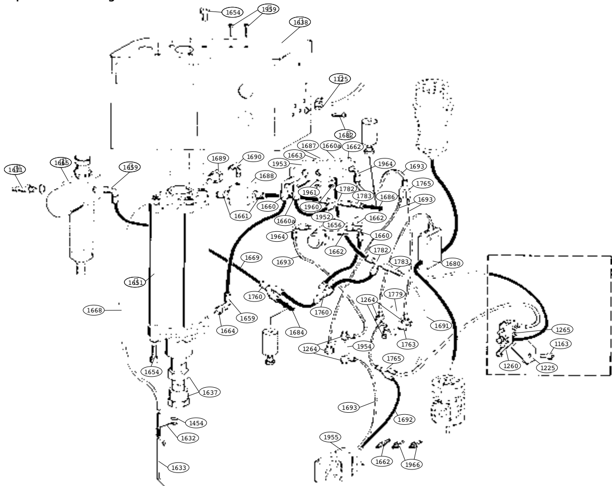
Abb. 41: Explosionszeichnung 4
