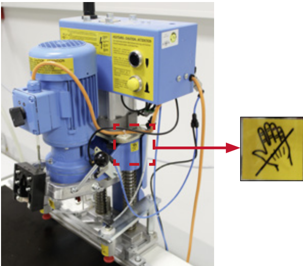
Abb. 9: Kennzeichnung – Gesamtmaschine
