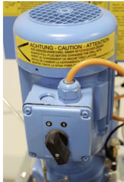
Abb. 12: Kennzeichnung – Motor/Antrieb
