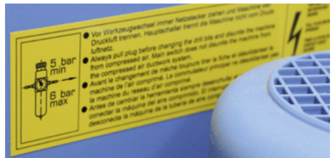
Abb. 13: Kennzeichnung – Gesamtmaschine
